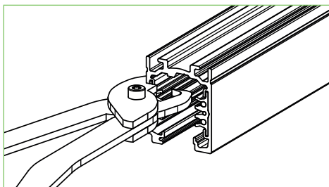
Abb. 4 Kürzen der Leiter Pic. 4 Reccessing track conductors
