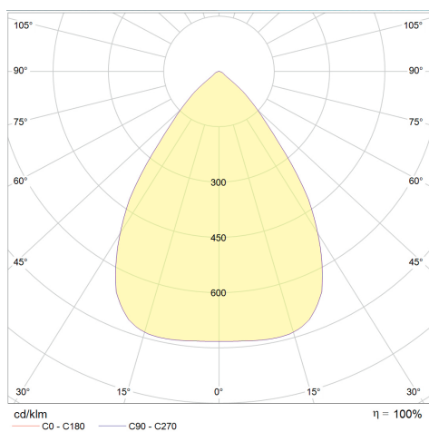
Polardiagramm 840, 73°
