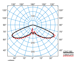
Publisca P1-RB6L/2600-730 3G1S
