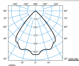
InperlaLP C05 HR22 IP 1800-830 ET 01
