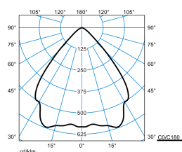
InperlaLP C05 HR22 IP 1800-830 01 + RD-PC
