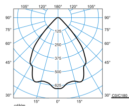
InperlaLP C05 HR22 IP 1800-830 01 + DA-M 01
