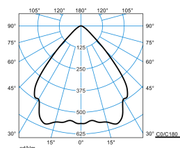
InperlaLP C05 HR22 IP 1800-830 01 + DA 01
