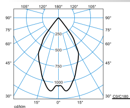
InperlaLP C05 BR22 2700-840 ET 03
