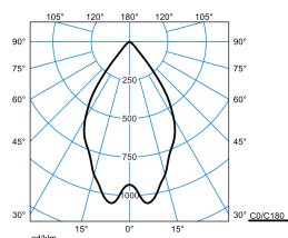
InperlaLP C05 BR22 2700-840 03 + DA 03
