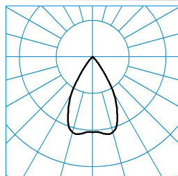
SNS RD5-HR1VFL-20-840
