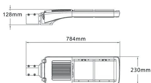
Abmessungen MAIN 120
