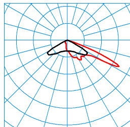
LnPlus 60-AM19L-SLR1/20000-740 16G1 ET (CLO initial value) TX376973
