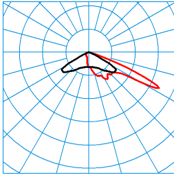
LnPlus 70-AM19L/42000-740 56G1 ETDD (CLO end value) TX377740
