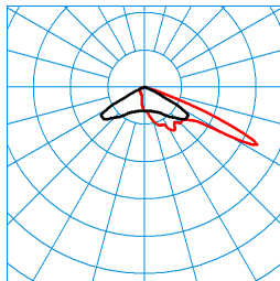
LnPlus 70-AM19L/38000-730 36G1 ETDD (CLO end value) TX390181
