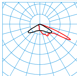
LnPlus 70-AM19L-LR/51000-730 48G1 ET (CLO end value) TX377306 DIN 5040: A30 UTE: 1,00 J CEN Flux Code: 28 76 99 100 100 ■ C0 - C180 ■ C90 - C270
