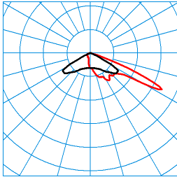
LnPlus 70-AM19L-SLR1/62000-730 48G1 ET (CLO initial value) TX377069
