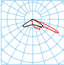
LnPlus 70-AM19L-SLR1/42000-730 36G1 ET (CLO end value) TX377166
