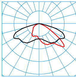
LnPlus 60-AB7L-SLR2/26000-730 24G1 ET (CLO end value) TX3900165
