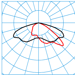
LnPlus 60-AB7L-SLR2/26000-730 24G1 ET (CLO initial value) TX3900096
