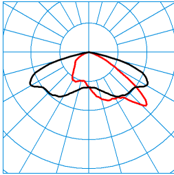
LnPlus 60-AB7L-LR/26000-727 24G1 ET (CLO end value) TX390135 ■ C0 - C180 ■ C90 - C270 DIN 5040: A30 UTE: 1,00 G CEN Flux Code: 35 73 98 100 100
