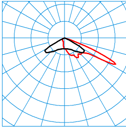
LnPlus 60-AM19L-SLR1/26000-722 24G1 ET (CLO initial value) TX390118
