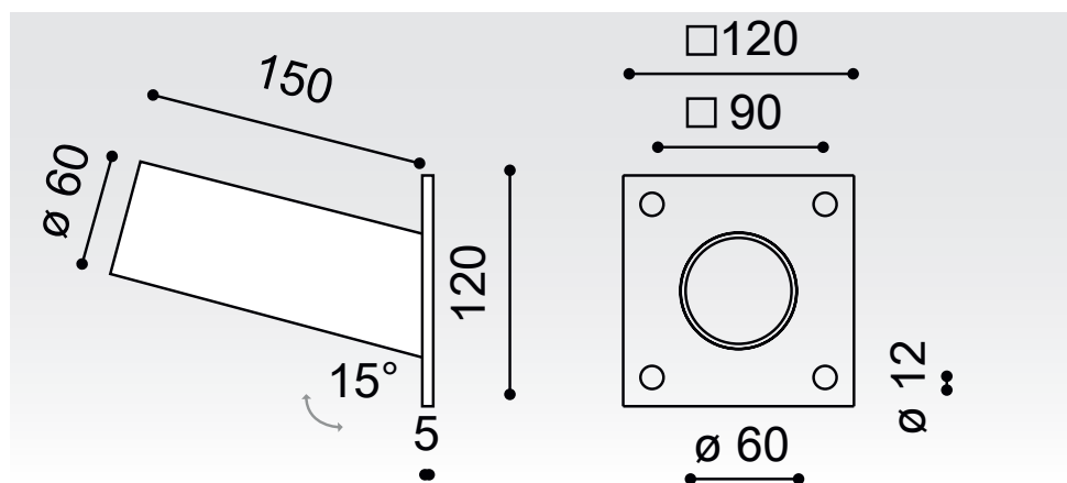
15° Wandhalterung
