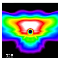
asymmetrisch breitstrahlend Höhe: 4,50m; Fläche: 30m x 30m
