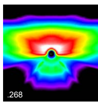
eng- und breitstrahlend Höhe: 4,50m; Fläche: 30m x 30m
