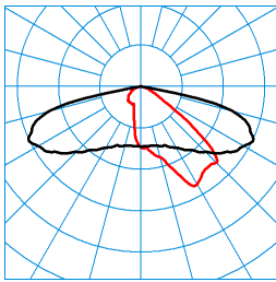
LIQ 50N-AB2L-LRA/4600-722 6G1 (CLO end value) TX281106 ■ C0 - C180 ■ C90 - C270 DIN 5040: A30 UTE: 1,00 G CEN Flux Code: 34 71 96 100 100 0 0 0 0
