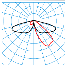
8841LS-Ü 360-AB2L/1000-730 2G2 ET (CLOANFANGSWERT) TX369394 ■ C0 - C180 ■ C90 - C270 DIN 5040: A20 UTE: 0,92 l + 0,08 T CEN Flux Code: 29 64 91 92 100 12 33 60 8
