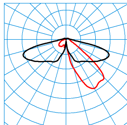
8841LS-Ü 360-AB2L/1000-730 2G2 ET (CLOENDWERT) TX369485 ■ C0 - C180 ■ C90 - C270 DIN 5040: A20 UTE: 0,92 l + 0,08 T CEN Flux Code: 29 64 91 92 100 12 33 60 8
