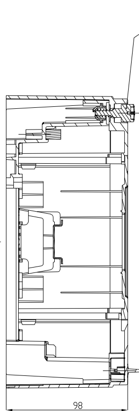
SNITT A-A
