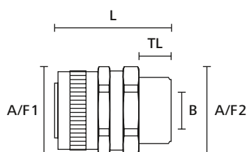
HelaGuard Verschraubung, gerade mit drehendem Außengewinde
