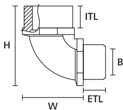
HelaGuard 90° Anschlusswinkel
