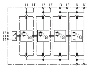
Prinzipschaltbild DV M TT 255 FM
