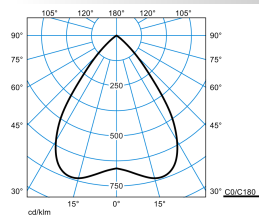
InperlaL G2 C07 BR19 1800-840 ET 01
