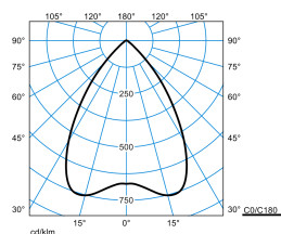
InperlaL G2 C07 BR19 1800-840 01 + RD-PC
