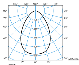
InperlaL G2 C07 BR19 1800-840 01 + DA-M 01
