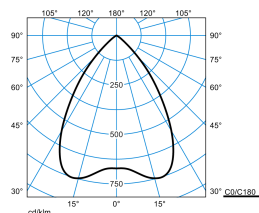
InperlaL G2 C07 BR19 1800-840 01 + DA 01
