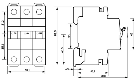
Maßzeichnung Gruppenansicht
