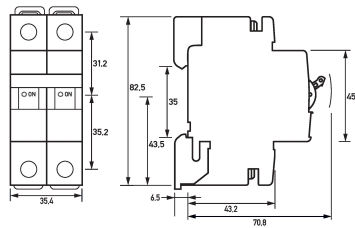
Maßzeichnung Gruppenansicht
