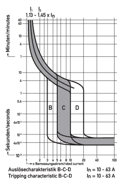
Diagramme Leitungsschutzschalter DLS 6i C63-3
