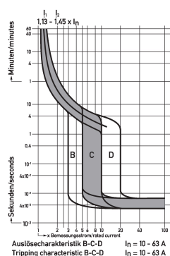
Diagramme Leitungsschutzschalter DLS 6i B63-1
