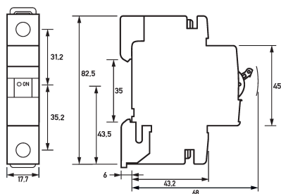
Maßzeichnung Leitungsschutzschalter DLS 6i B63-1
