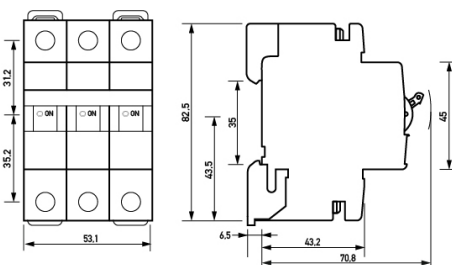
Maßzeichnung Gruppenansicht
