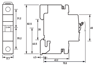
Maßzeichnung Gruppenansicht
