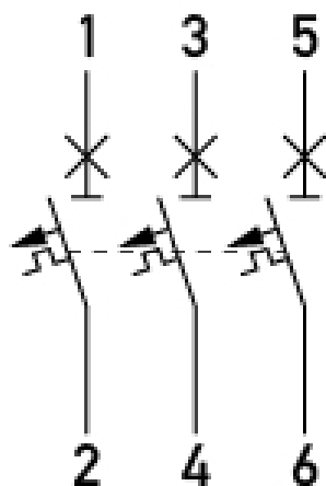
Anschlusschema
