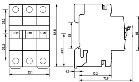
Maßzeichnung Gruppenansicht
