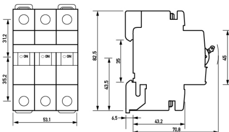
Maßzeichnung Gruppenansicht
