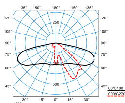
Publisca P2-AB2L-LR/1500-740 2G1S
