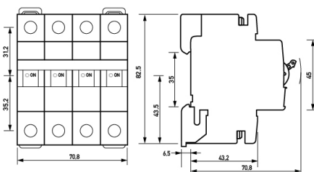
Maßzeichnung Gruppenansicht
