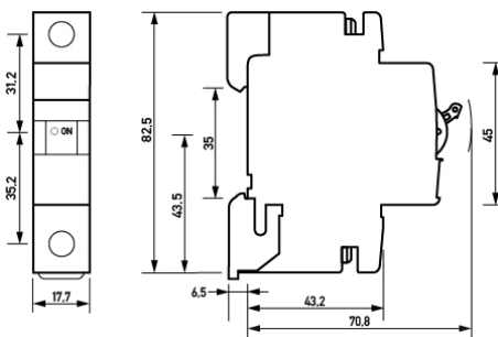
Maßzeichnung Gruppenansicht
