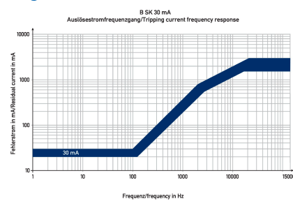
Kennlinie B SK 30 mA
