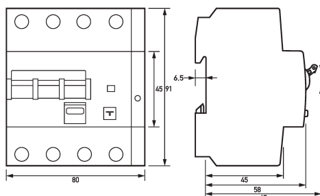
Maßzeichnung FI-/LS-Kombinationen DRCBO 4 C32/0,10/3N-B SK
