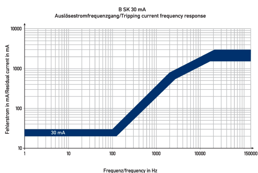
Diagramme FI-/LS-Kombinationen DRCBO 4 C32/0,03/1N-B SK
