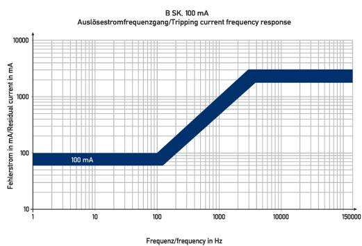
Diagramme FI-/LS-Kombinationen DRCBO 4 C25/0,10/1N-B SK
