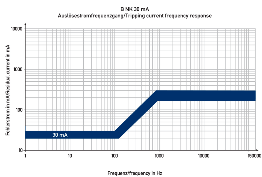
Diagramme FI-/LS-Kombinationen DRCBO 4 C25/0,03/3N-B NK
