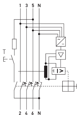
Schaltungsbeispiel FI-/LS-Kombinationen DRCBO 4 C25/0,03/3N-B NK
