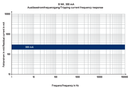
Diagramme FI-/LS-Kombinationen DRCBO 4 C20/0,30/1N-B NK
