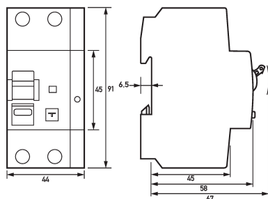
Maßzeichnung FI-/LS-Kombinationen DRCBO 4 C20/0,30/1N-B NK
