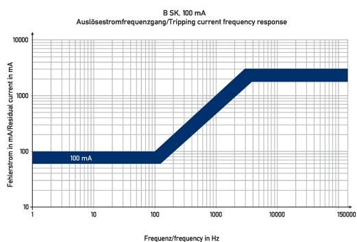
Diagramme FI-/LS-Kombinationen DRCBO 4 C20/0,10/3N-B SK
