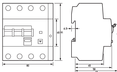
Maßzeichnung FI-/LS-Kombinationen DRCBO 4 C20/0,10/3N-B SK
