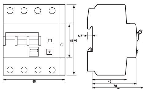
Maßzeichnung FI-/LS-Kombinationen DRCBO 4 C20/0,10/3N-B+
