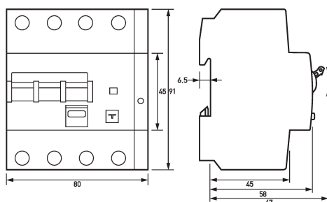
Maßzeichnung FI-/LS-Kombinationen DRCBO 4 C16/0,10/3N-B SK
