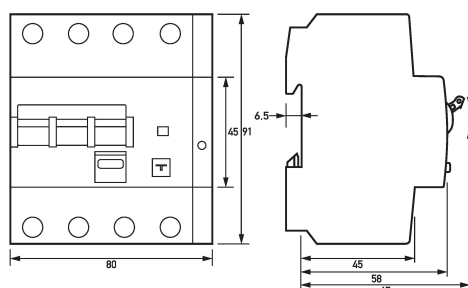
Maßzeichnung FI-/LS-Kombinationen DRCBO 4 C13/0,10/3N-B SK
