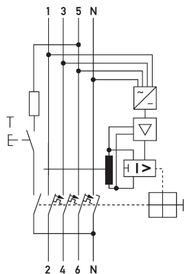
Schaltungsbeispiel FI-/LS-Kombinationen DRCBO 4 C13/0,10/3N-B+
