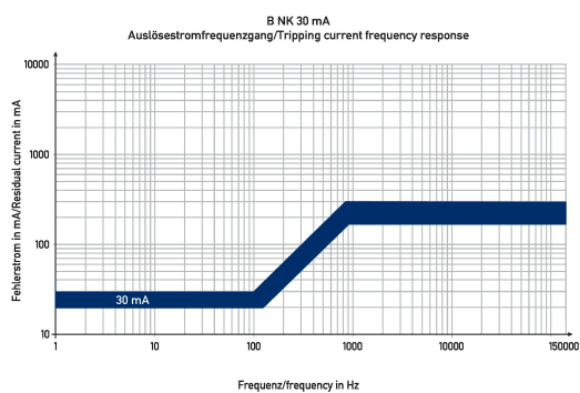
Diagramme FI-/LS-Kombinationen DRCBO 4 C10/0,03/3N-B NK
