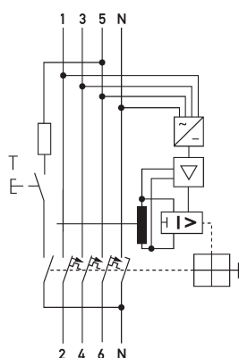
Schaltungsbeispiel FI-/LS-Kombinationen DRCBO 4 C10/0,03/3N-B NK
