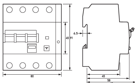
Maßzeichnung Gruppenansicht
