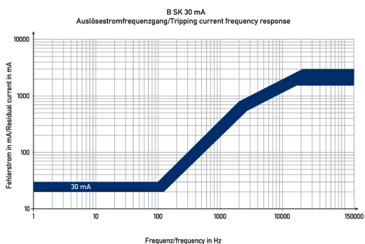
Diagramme FI-/LS-Kombinationen DRCBO 4 Co6/0,03/3N-B SK
